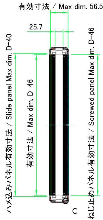
B-B ( 1 : 7 )
